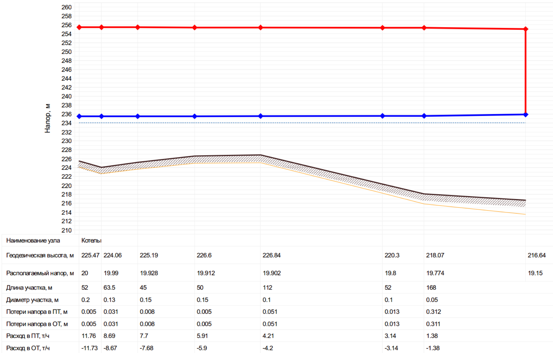
Рисунок 7 - Пьезометрический график тепловой сети от котельной №2 (р.п. им. В.И. Ленина, ул. Молодежная, 3а) до определяющего потребителя – жилой дом (р.п. им. В.И. Ленина, ул. Молодежная, 9)
