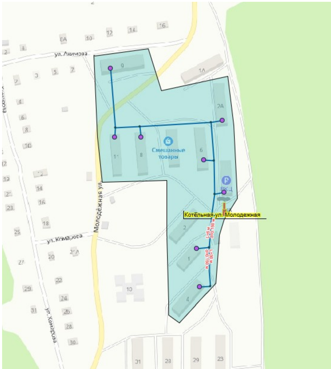
Рисунок 5 – Зона действия источников теплоснабжения р.п. им. В.И. Ленина (Котельная №2 (р.п. им. В.И. Ленина, ул. Молодёжная, 3а))
